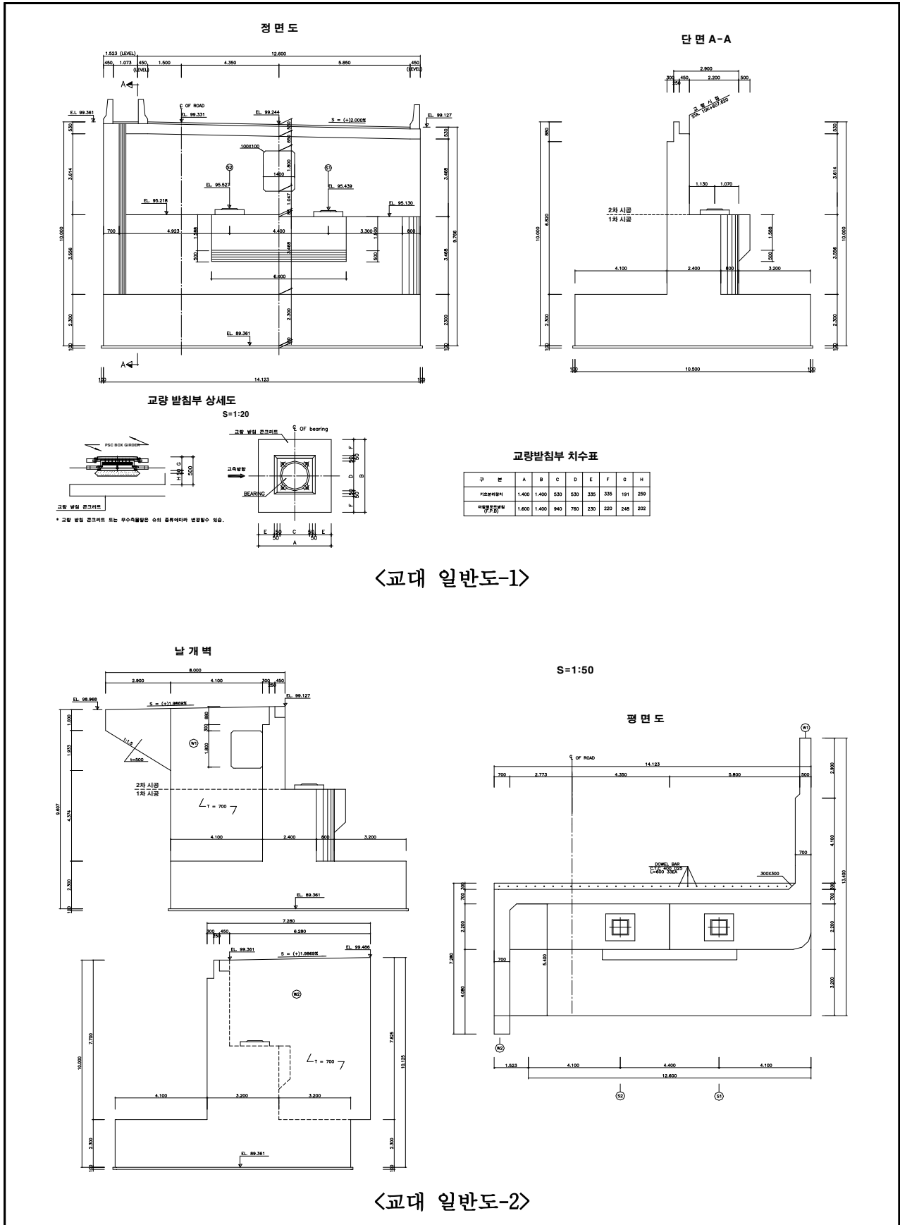
【그림 1.4.9】 남천대교(부산) 교대 일반도
