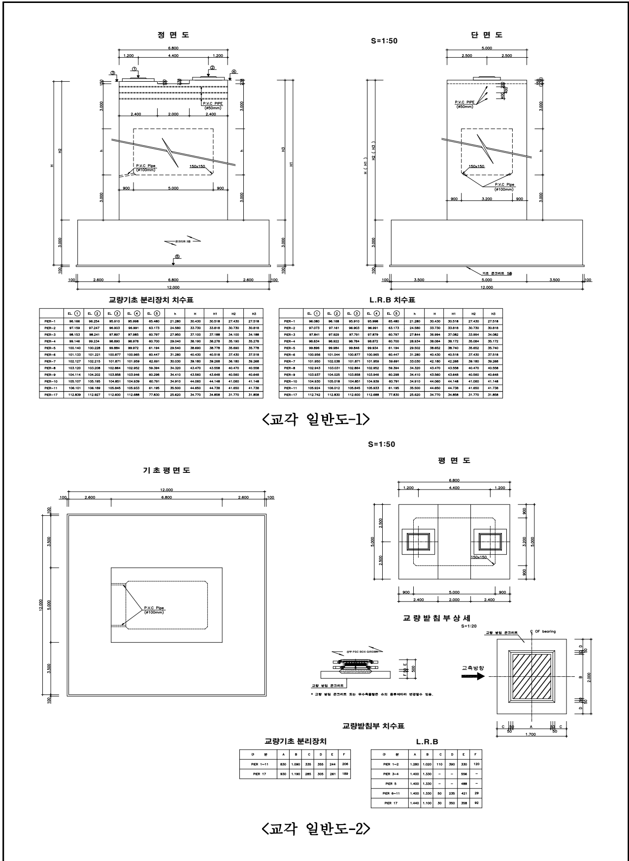
【그림 1.4.5】 남천대교(대구) 교각 일반도
